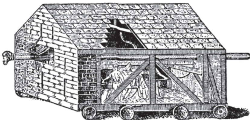
Эллинистическая военная техника. Таран на колёсах.
